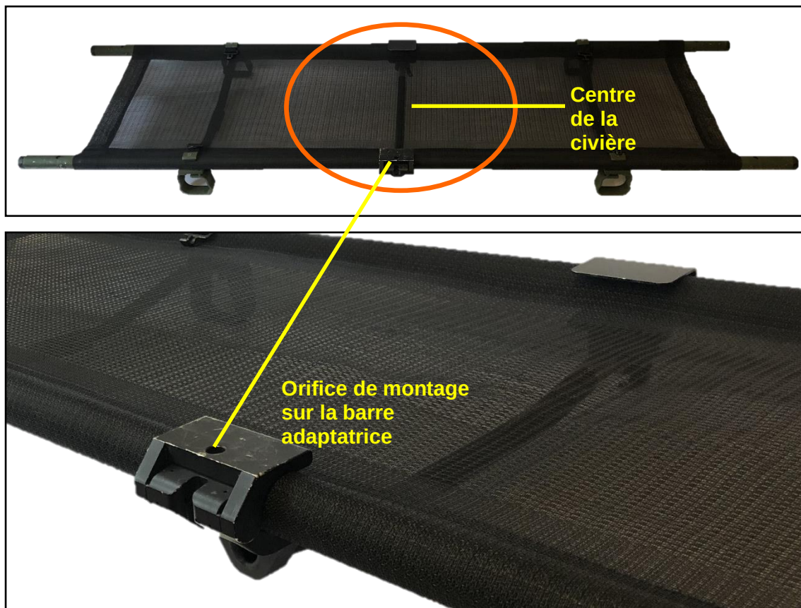
Illustration 9-4 : Barre adaptatrice de civière pour l'appareil MOVES® SLC™ installée sur une civière
