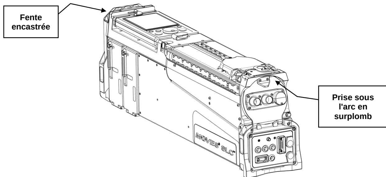
Illustration 9-1 : Emplacement des prises pour soulever l'appareil MOVES® SLC™
