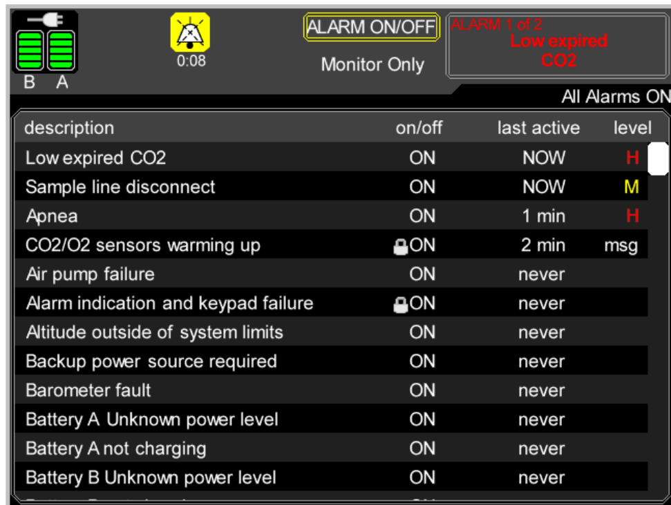
Illustration 11-28 : Écran Alarm On/Off (alarme activée/désactivée)
